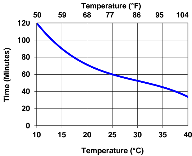
Interline 925: Pot Life
