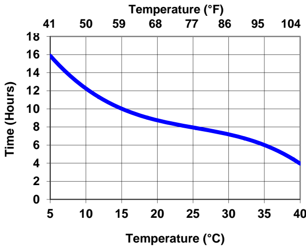
Interline 344: Pot Life
